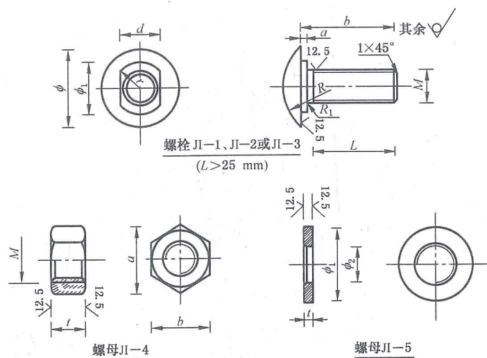
图 16 拼接螺栓
