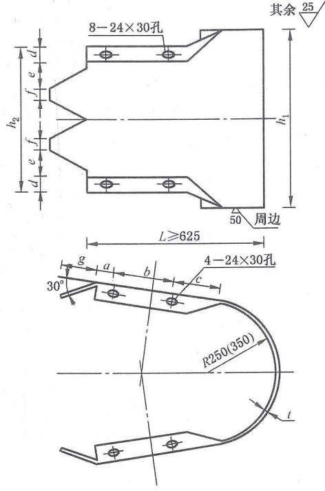
图 15 B型端头
