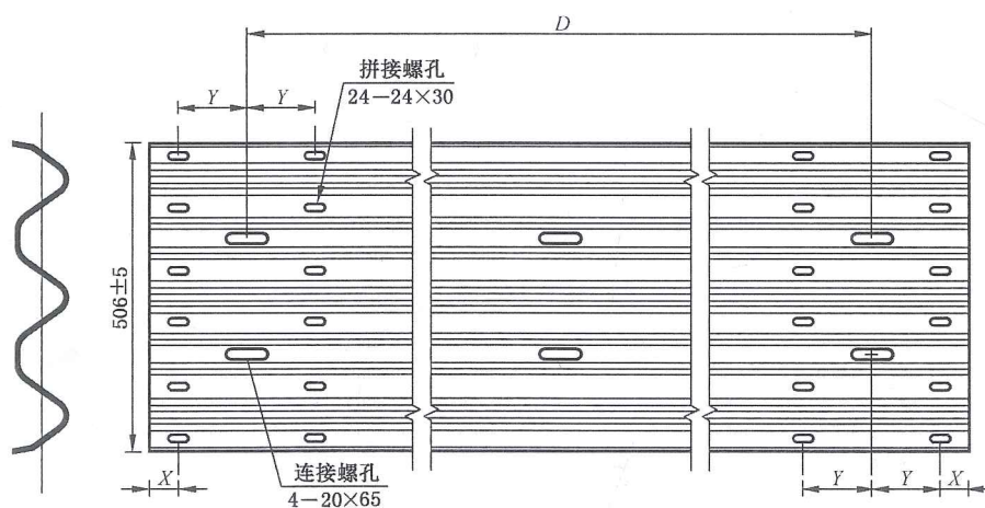
b) 钢管立柱或 H 型钢立柱用板
