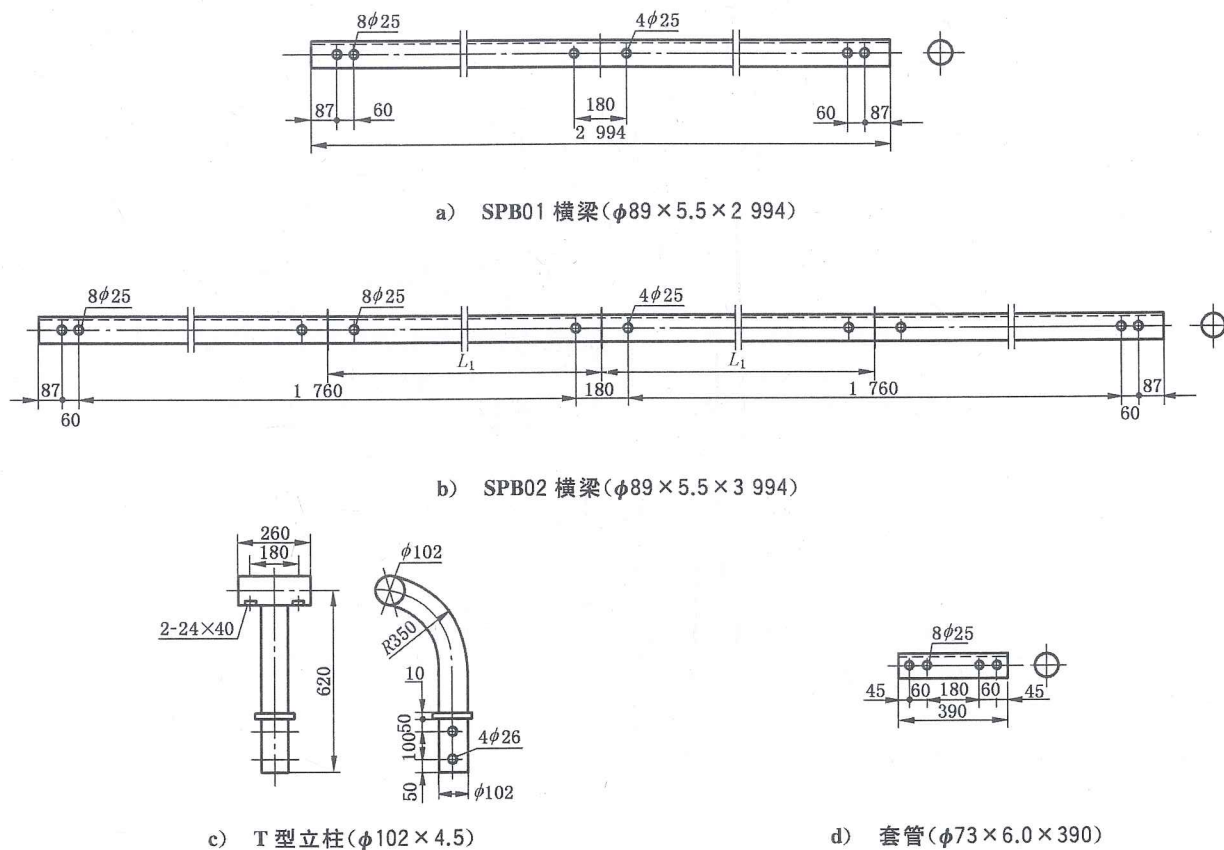
图 18 加强横梁
