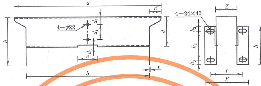
图 13 横隔梁
