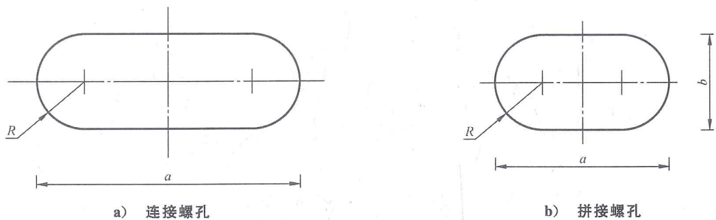
图 5 螺孔尺寸
