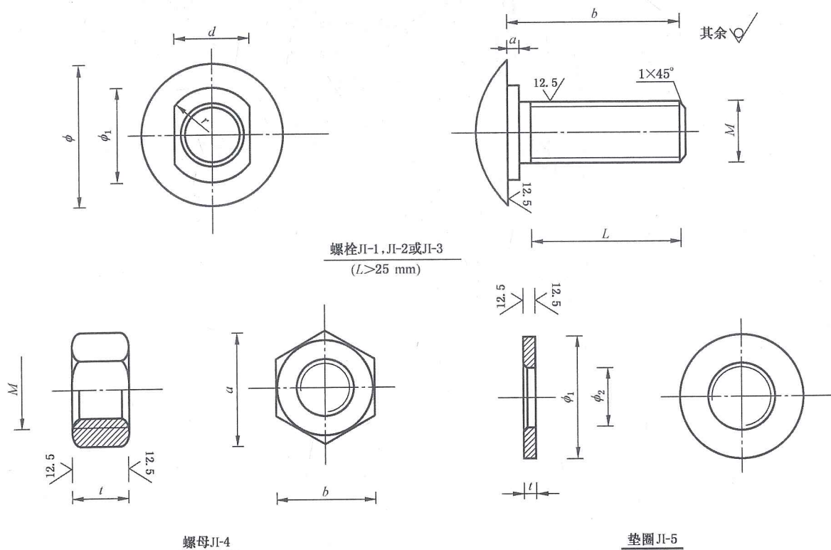
图 10 拼接螺栓
