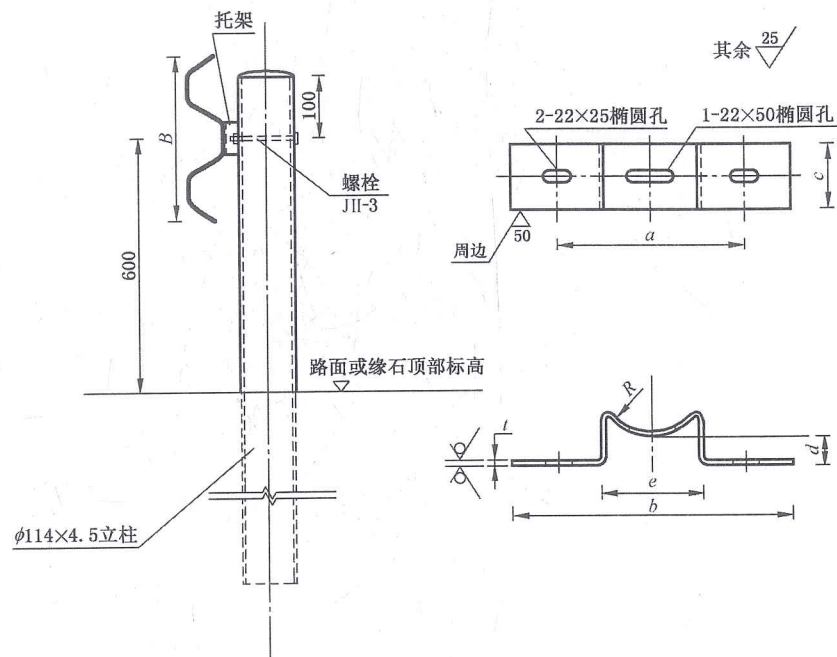
图 13 托架
