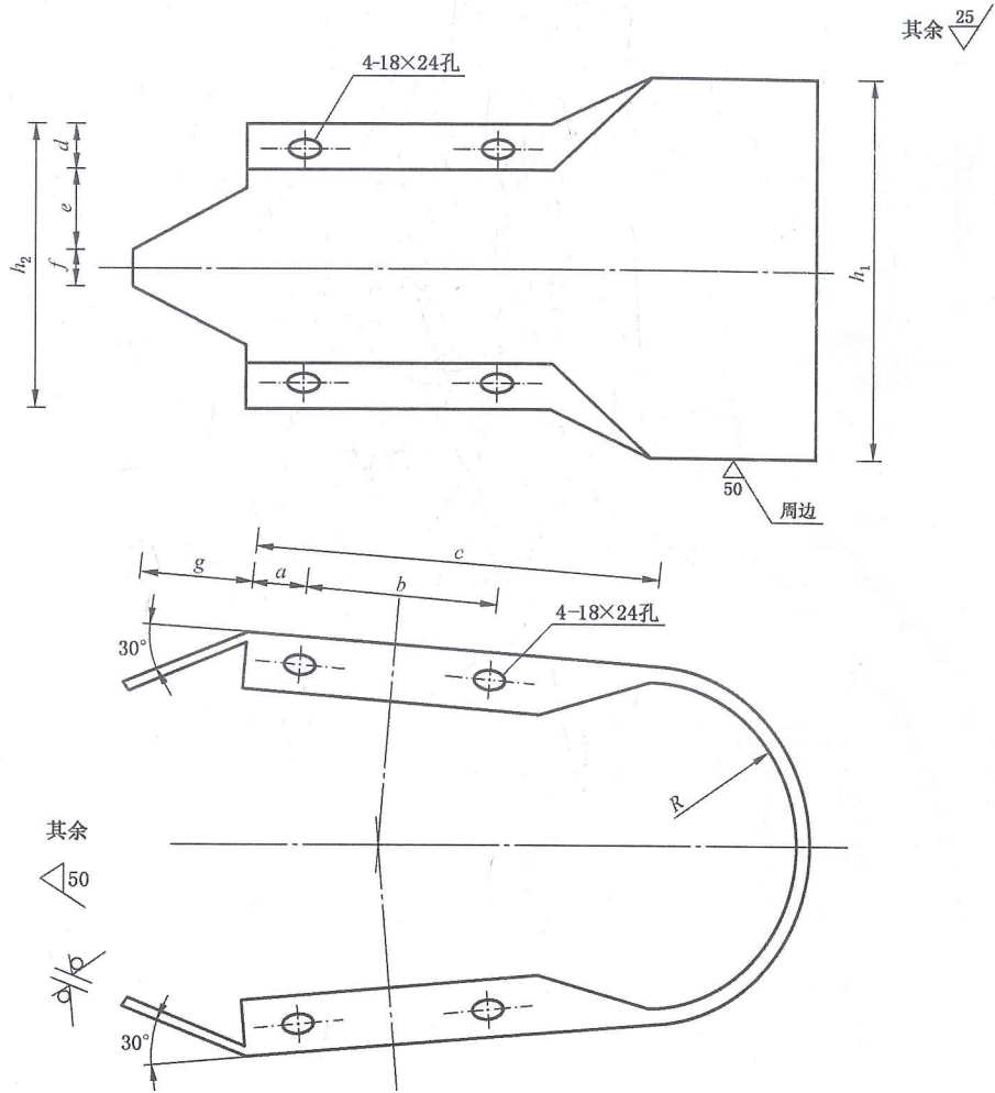
图 9 端头(D-II 或 D-III)
