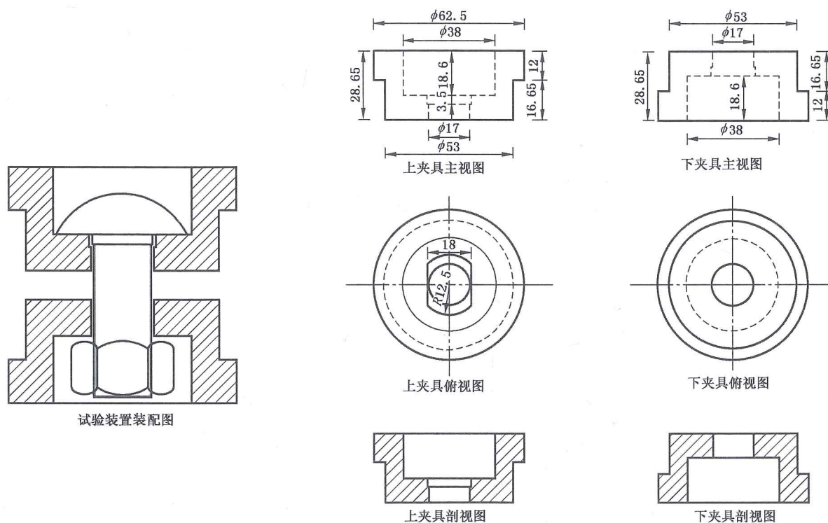
图 A.1 抗拉荷载试验装置图
