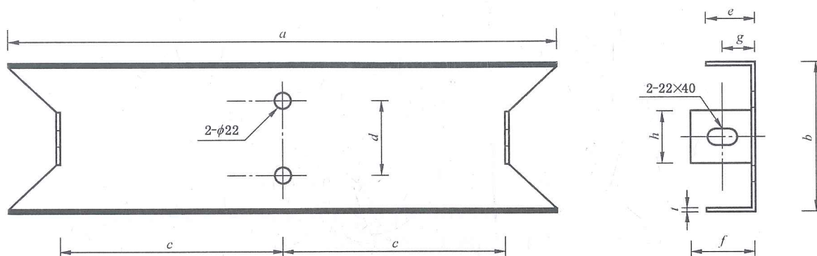
图 14 横隔梁
