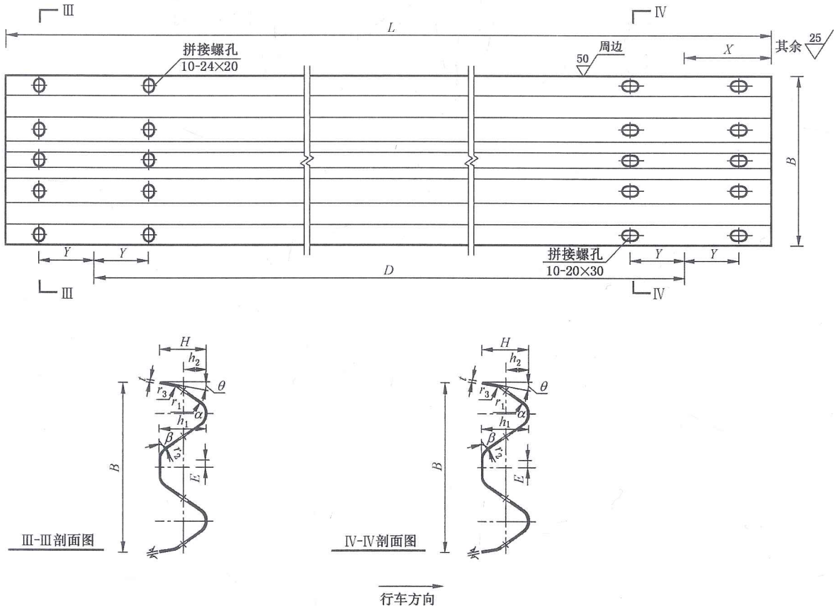
图 1 波形梁板(DB 类-1)
