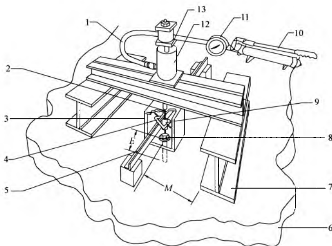
图 3.2.6 锚栓现场拉拔检测装置
