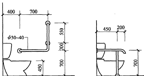
图 18 坐便器两侧固定式安全抓杆(mm)
