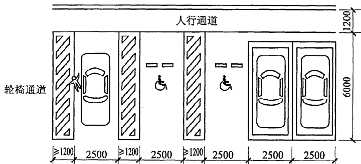
图 7 无障碍停车位及轮椅通道(mm)
