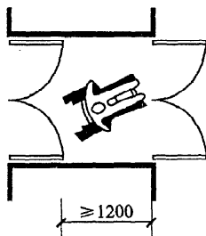
图 8 小型公建门厅门扇间距(mm)
