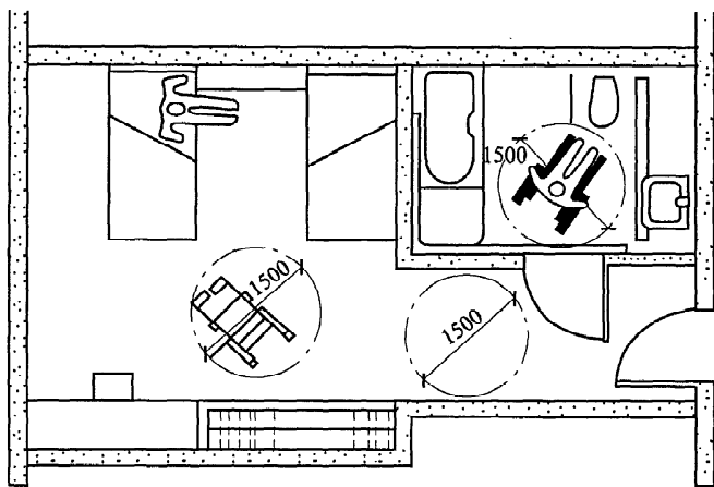
图 19 无障碍客房平面布置图(mm)
