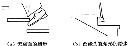
图 14 无踢面踏步和凸缘为直角形的踏步
