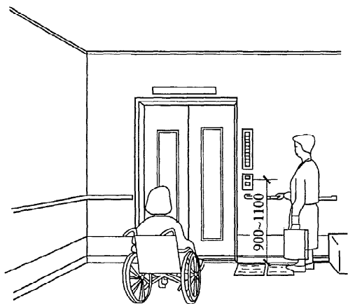
图 12 无障碍电梯候梯厅(mm)
