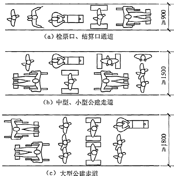
图 5 无障碍通道最小宽度(mm)
