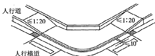
图 1 单面坡缘石坡道(mm)
