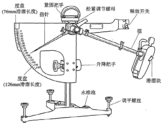
图 C. 0. 3 摆式仪结构示意图
