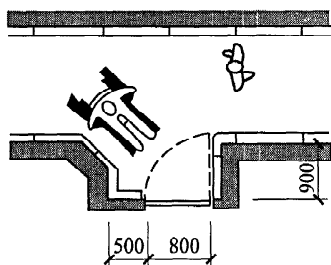
图 6 走道的凹室(mm)
