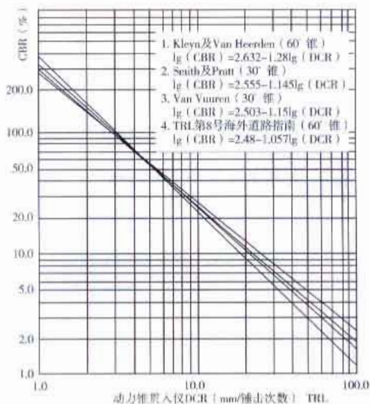
图 T 0045-2 DCR-CBR 关系图
