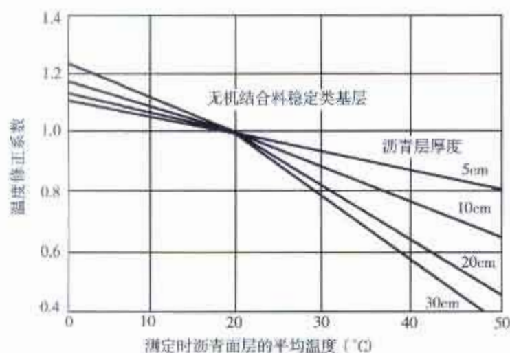
图 T 0951-4 路面弯沉温度修正系数曲线(适用于无机结合料稳定的半刚性基层)
