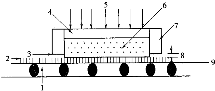
图 T 1129-1 接触面积不变直剪仪示意图
