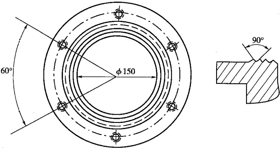
图 T 1126-1 夹持设备(尺寸单位:mm)
