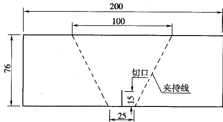
图 T 1125-1 梯形试样平面图(尺寸单位:mm)
