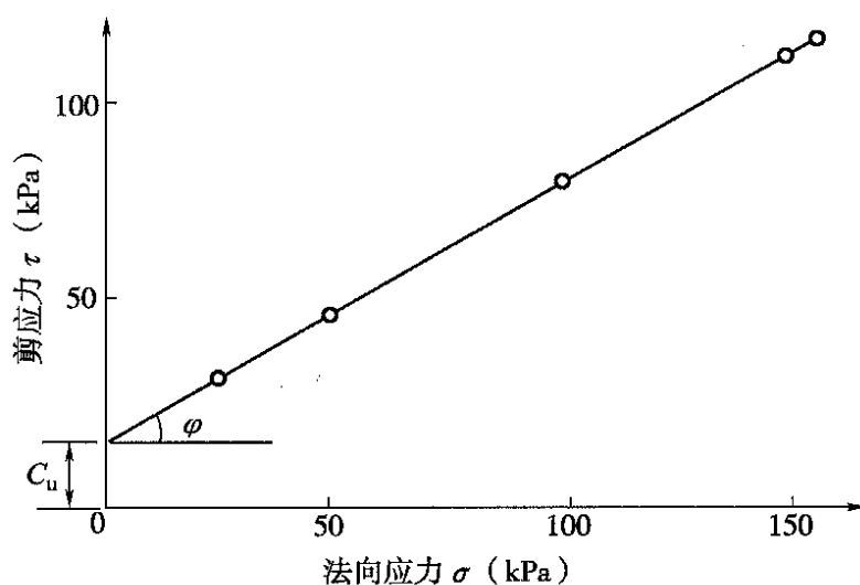
图 T 1130-3 \tau - \sigma 曲线
