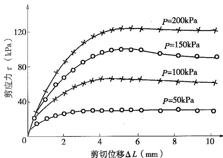
图 T 1129-3 剪应力与位移关系曲线
