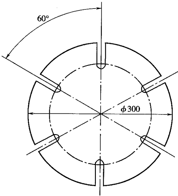
图 T 1126-3 试样(尺寸单位:mm)
