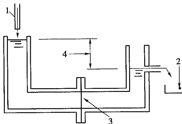
图 T 1141-1 水平式恒水头渗透仪示意图 1-进水系统;2-出水收集;3-试样;4-水头差
