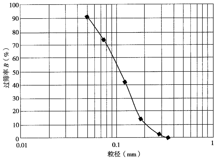
图 T 1144-1 有效孔径分布曲线
