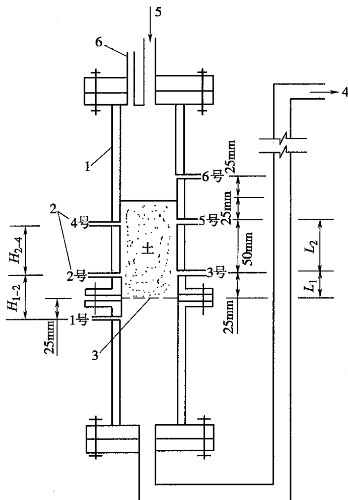
图 T 1145-1 梯度比装置示意图
