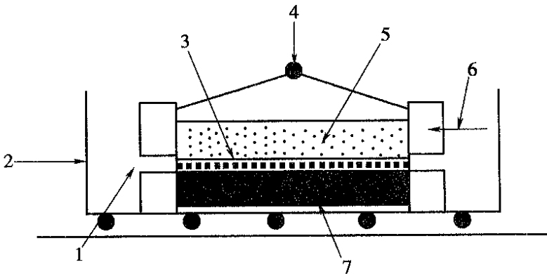
图 T 1129-2 接触面积递减直剪仪示意图
