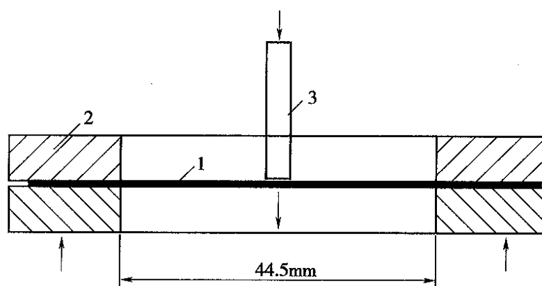
图 T 1127-1 刺破试验示意图
