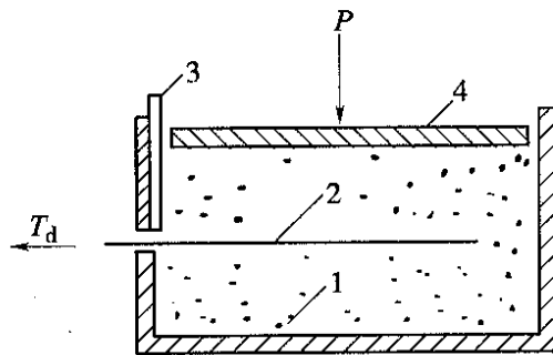
图 T 1130-1 拉拔试验箱示意图
