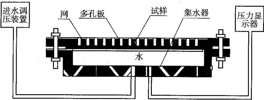
图 T 1142-1 耐静水压装置示意图
