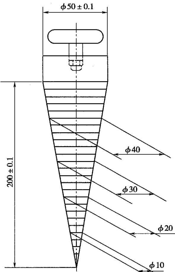
图 T 1128-2 量锥示意图(尺寸单位:mm)
