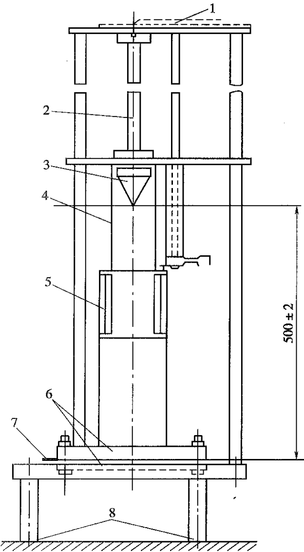
图 T 1128-1 落锥架示意图(尺寸单位:mm)
