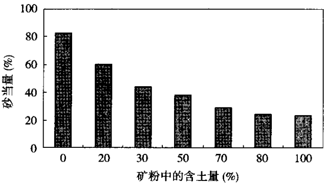
图 T0334-5 矿粉中土的含量对砂当量的影响
