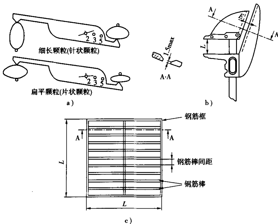
图 T0312-2 国外粗集料针片状颗粒含量测定仪示意图
