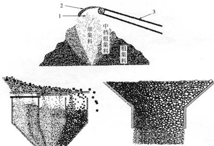
图 T0301-4 集料离析情况 1-细集料;2-粗集料;3-传送带
