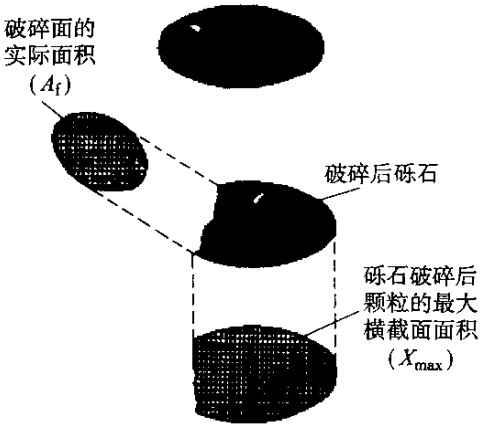
图 T0346-1 破碎面的定义
