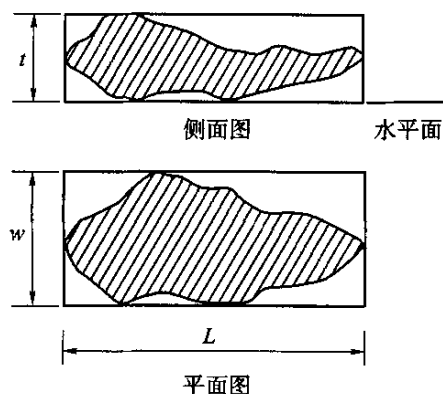
图 T0312-1 针片状颗粒稳定状态
