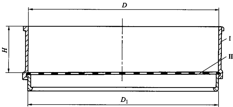
图 A-1 标准筛的筛框(I-筛框;II-筛面)
