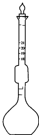
图 T0352-1 李氏比重瓶
