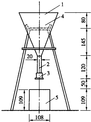
图 T0331-1 标准漏斗(尺寸单位:mm) 1-漏斗;2- \phi 20\text{mm} 管子;3-活动门;4-筛; 5-金属量筒
