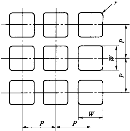
图 A-3 方孔筛金属穿孔板的式样 W-筛孔基本尺寸；P-孔中心距；r-圆角半径
