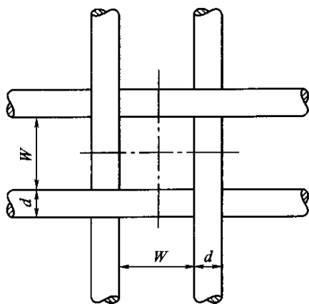
图 A-2 金属丝编织网的形状与要求 W-筛孔基本尺寸；d-金属丝直径
