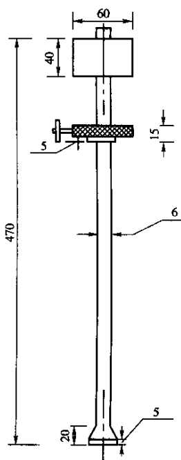
图 T0334-3 配重活塞 (尺寸单位: mm)
