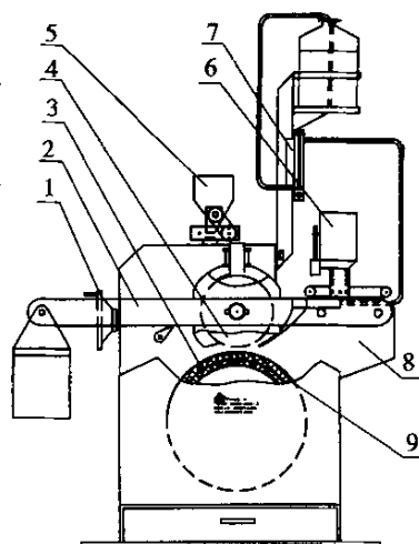
图 T0321-1 加速磨光试验机
