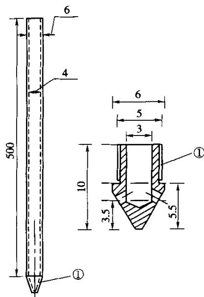
图 T0334-2 冲洗管(尺寸单位: mm)
