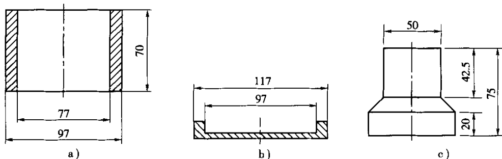
图 T0350-1 细集料压碎指标试模(尺寸单位:mm)
