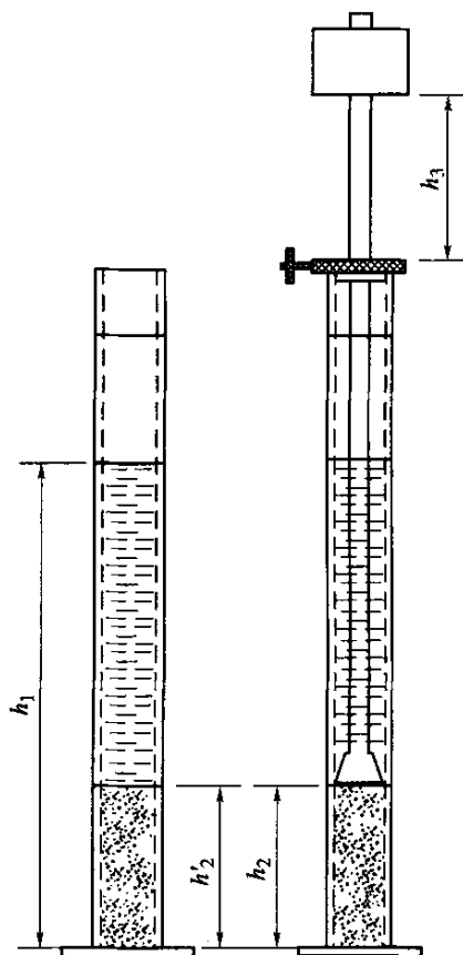
图 T0334-4 读数示意图
