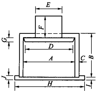
图 T0316-1 压碎指标值测定仪 (尺寸单位：mm)
