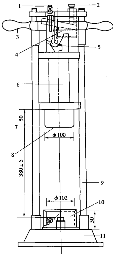
图 T0322-1 冲击试验仪 (尺寸单位: mm)
