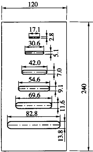
图 T0311-2 片状规范仪(尺寸单位:mm)
