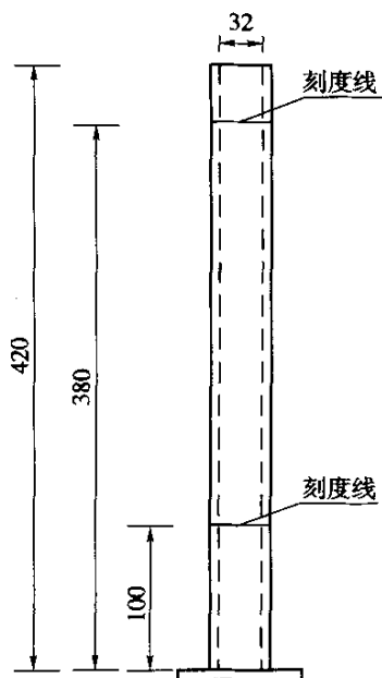
图 T0334-1 透明圆柱试筒(尺寸单位: mm)
