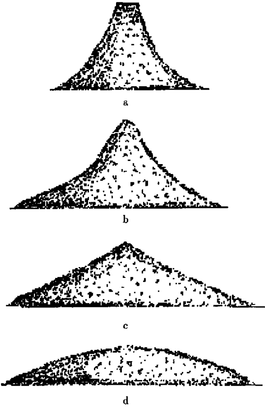
图 T0330-3 欧洲 CEN 标准 EN 933-6 及英国 BS 812 标准中的状态照片
