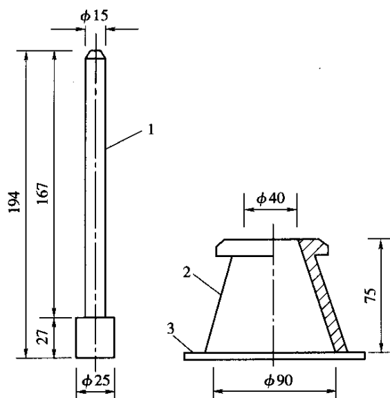
图 T0330-1 饱和面干试模及其捣棒(尺寸单位:mm)
