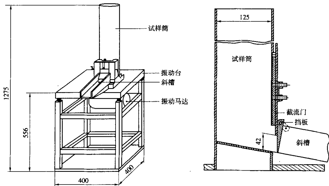
图 T0346-2 欧洲的粗集料棱角性测试仪(左为仪器全图,右为斜槽漏斗部分大样图,单位:mm)
