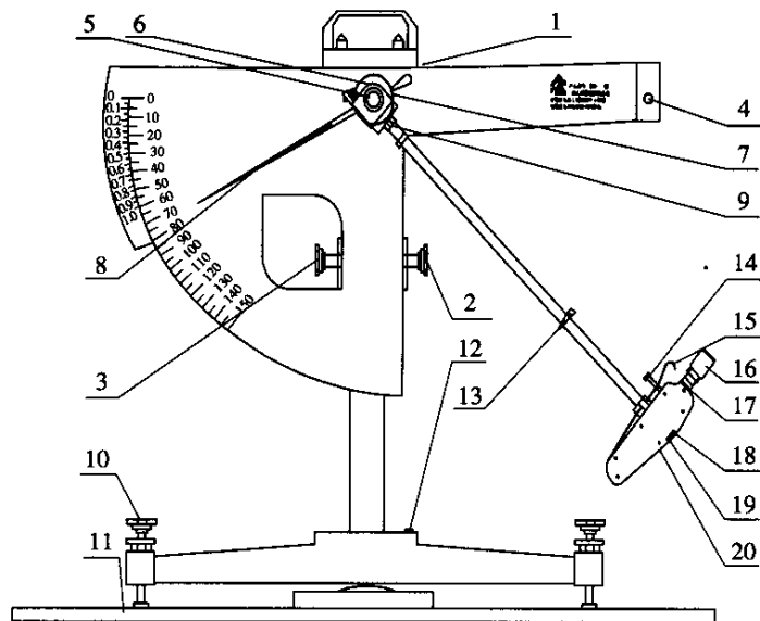
图 T0321-2 摆式摩擦系数测定仪
