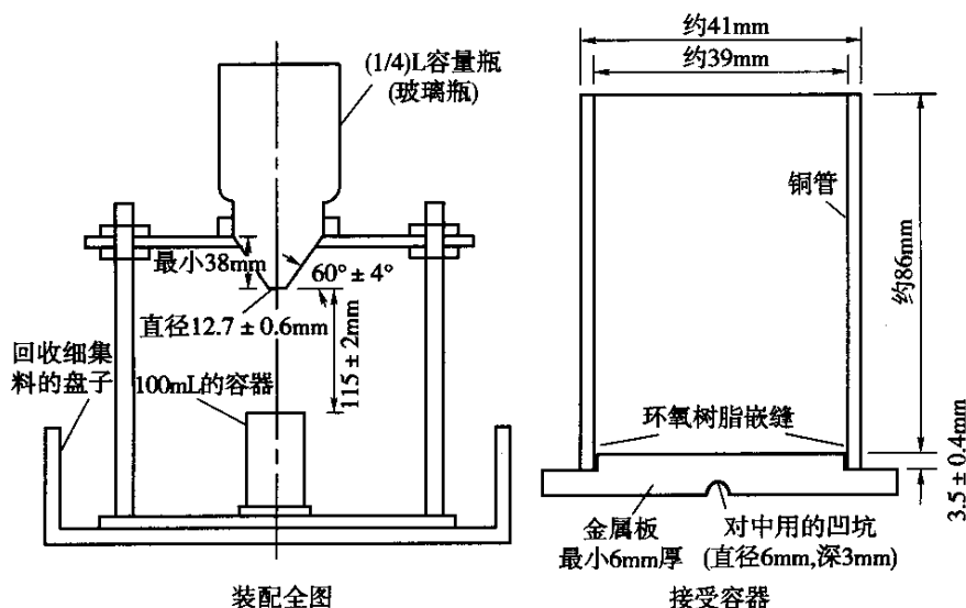
图 T0344-1 细集料棱角性测定装置
